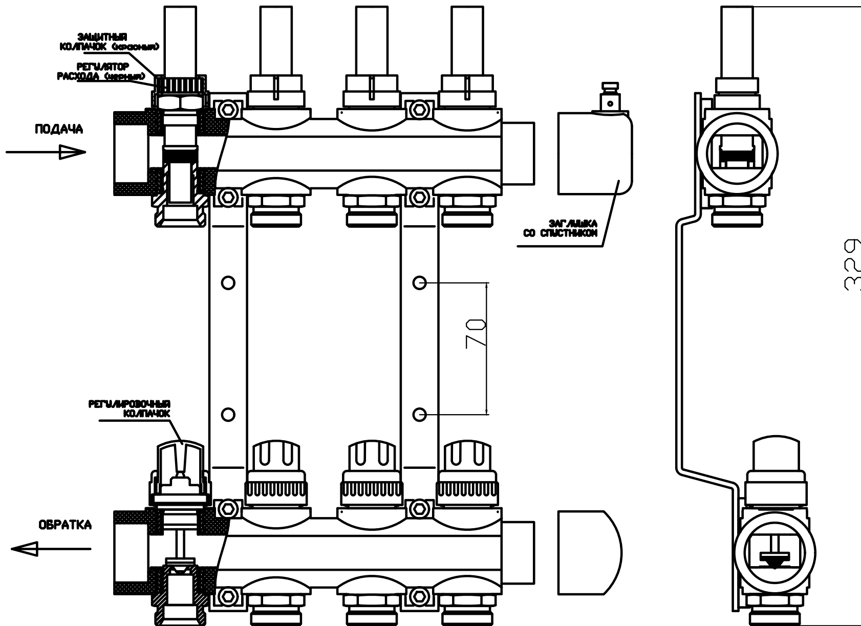
Рис 2. Пример сборки коллекторов (подвод и отвод слева)
