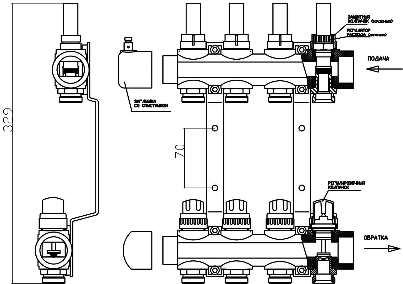
Рис 1. Пример сборки коллекторов (подвод и отвод справа)
